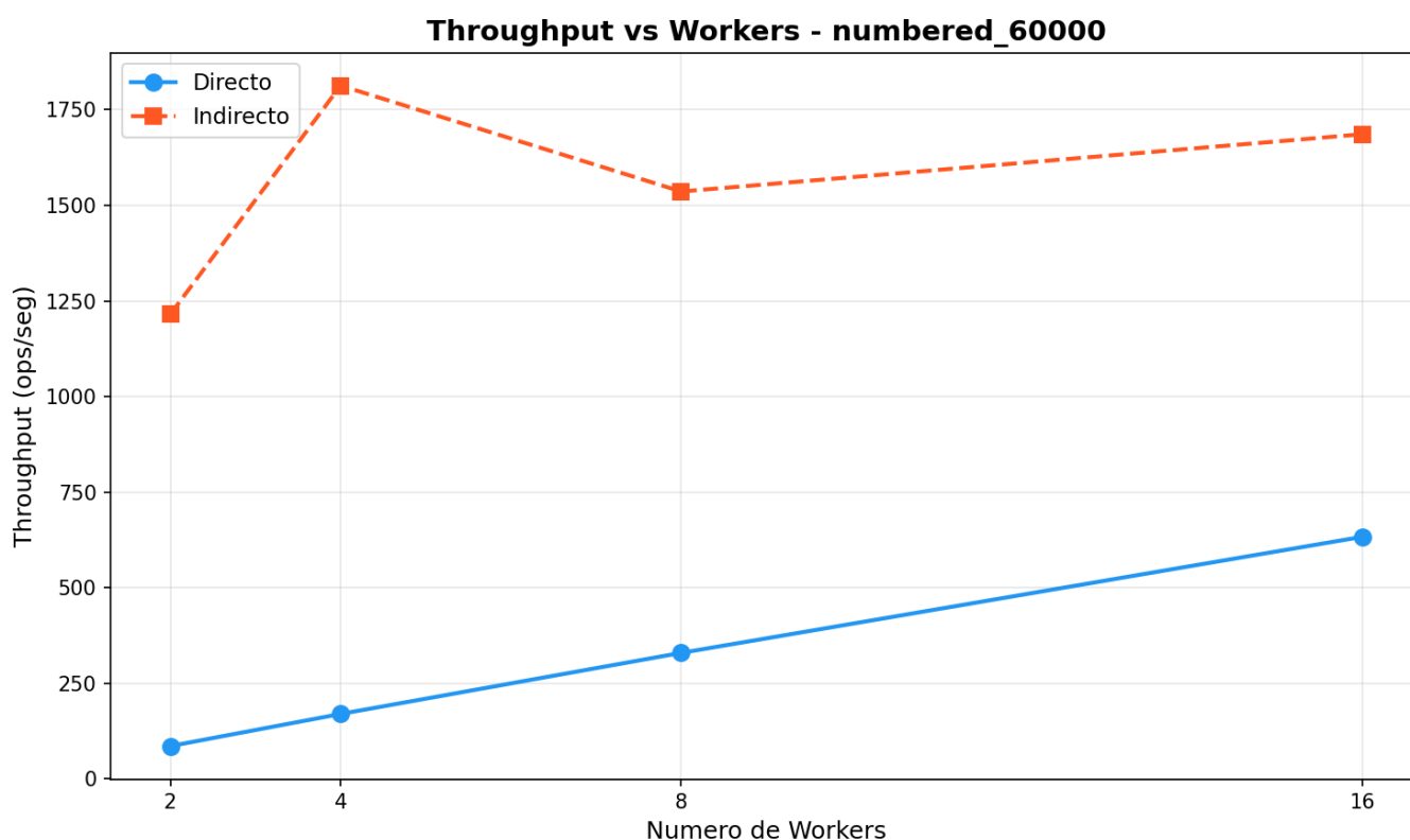
Fig. 5 - Throughput vs Workers (entradas numeradas, hotspot seat 42)
