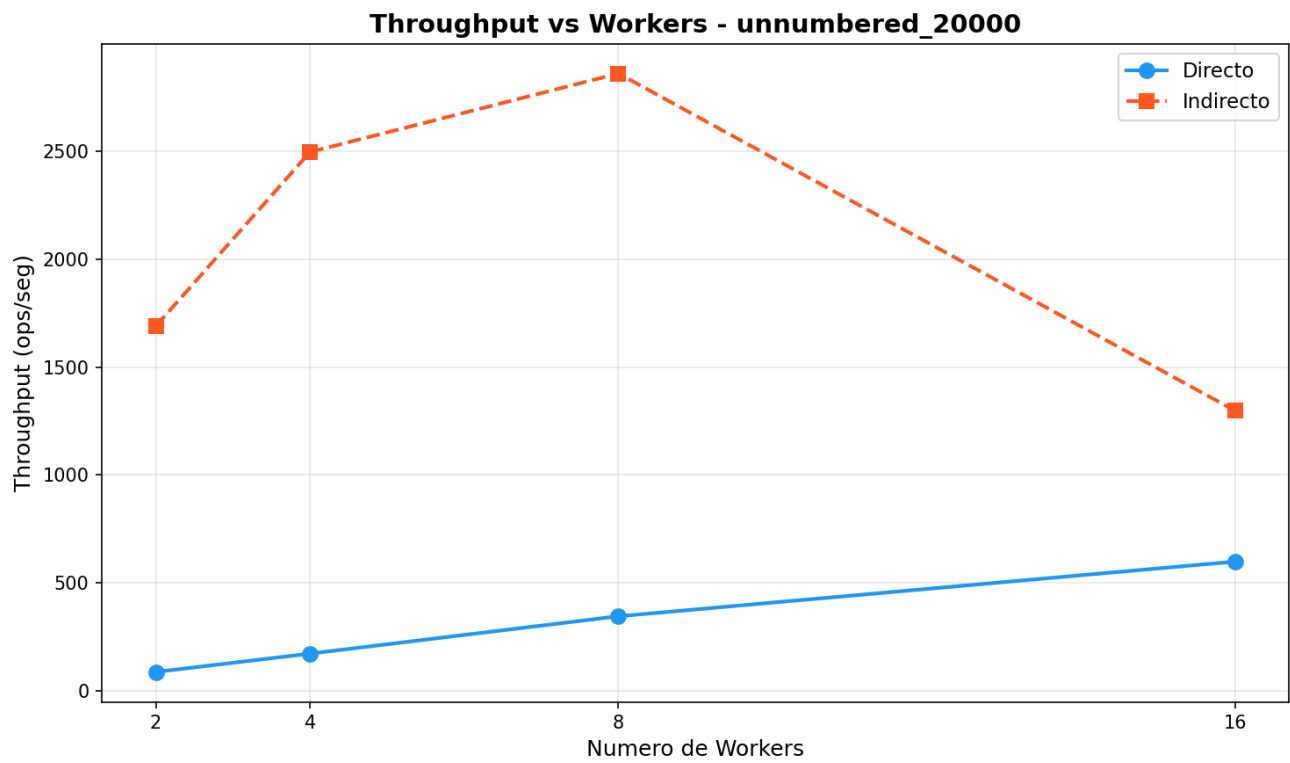
Fig. 4 - Throughput vs Workers (entradas no numeradas)
